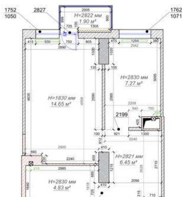
Обмерный план
